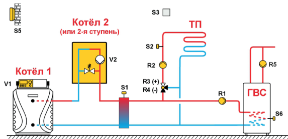
Схема шкафа управления М-Вох-12-4
