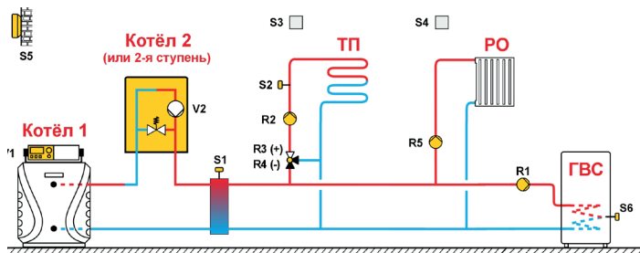
Схема шкафа управления М-Вох-12-2
