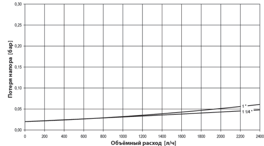
Рабочая диаграмма насосного модуля DK
