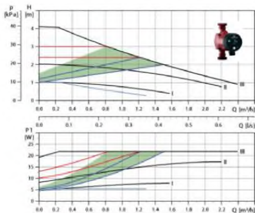
Рис.10: Характеристики насоса Alpha2 xx40
