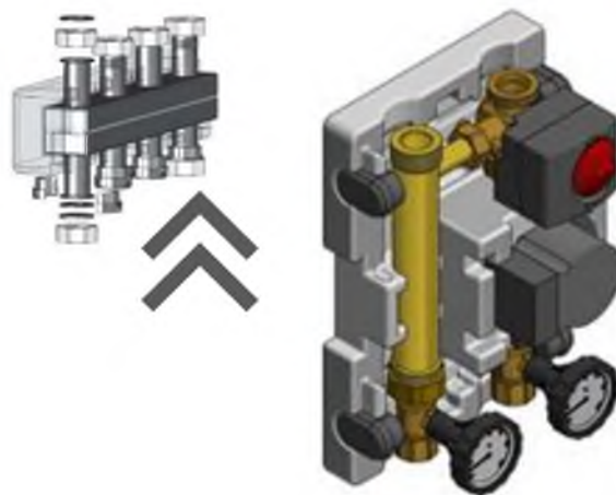
Рис.24: Насосная группа DN25 - Повышение температуры обратной линии
