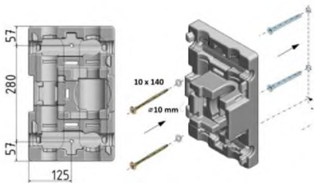
Рис.4: Настенное крепление насосных групп
